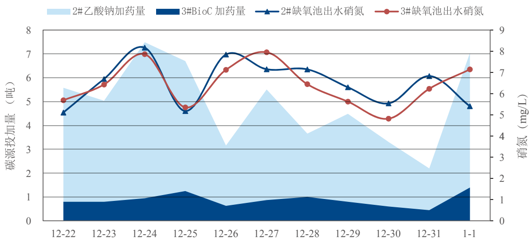
碳源对比投加缺氧池出水硝氮的变化
