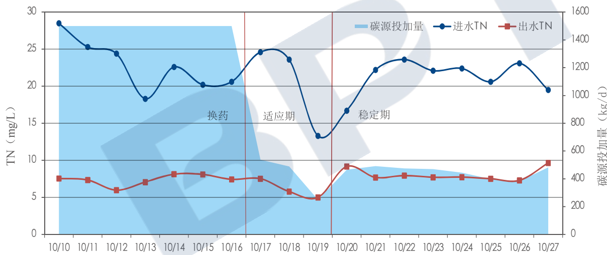
投加BioC-1M碳源后系统出水TN的对比结果分析
