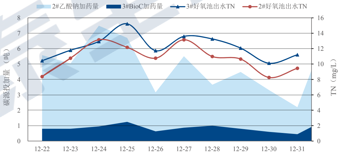
碳源对比投加好氧池出水TN的变化
